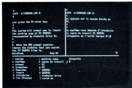
Exemple d'écran obtenu avec le système d'aide à la traduction ALPS, sur IBM PC.
