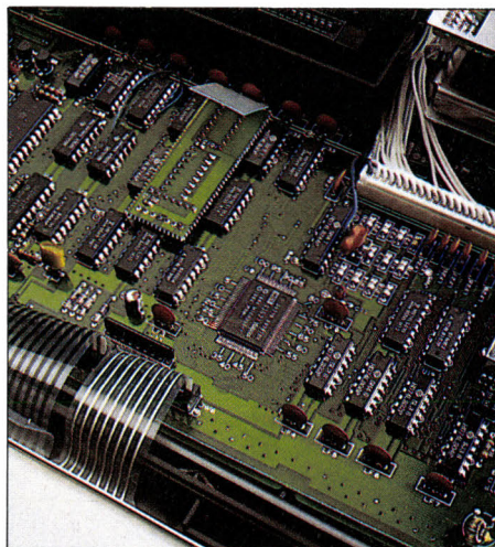
Au centre, le boîtier à 100 broches du MSX System, cœur logique de la machine.
