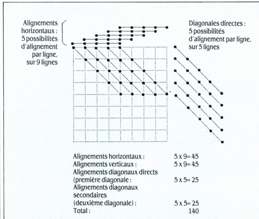
Figure 2. Sur un terrain 9x9, il y a exactement 140 alignements possibles de 5 pions. Au cours de l'initialisation, le programme en construit une liste qu'il utilise pour évaluer la position.
