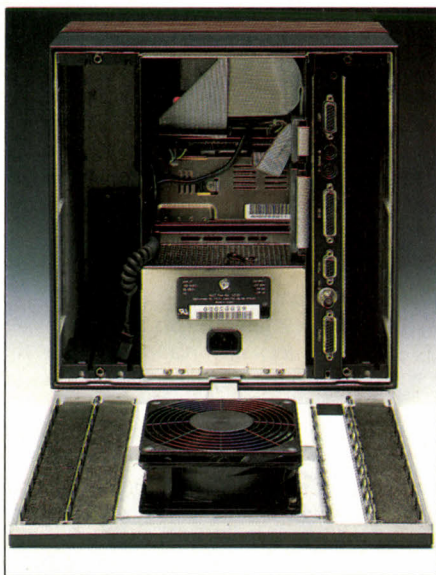
À l'intérieur du Next, toute l'électronique est regroupée sur une seule carte, laissant la place pour trois cartes d'extension.
