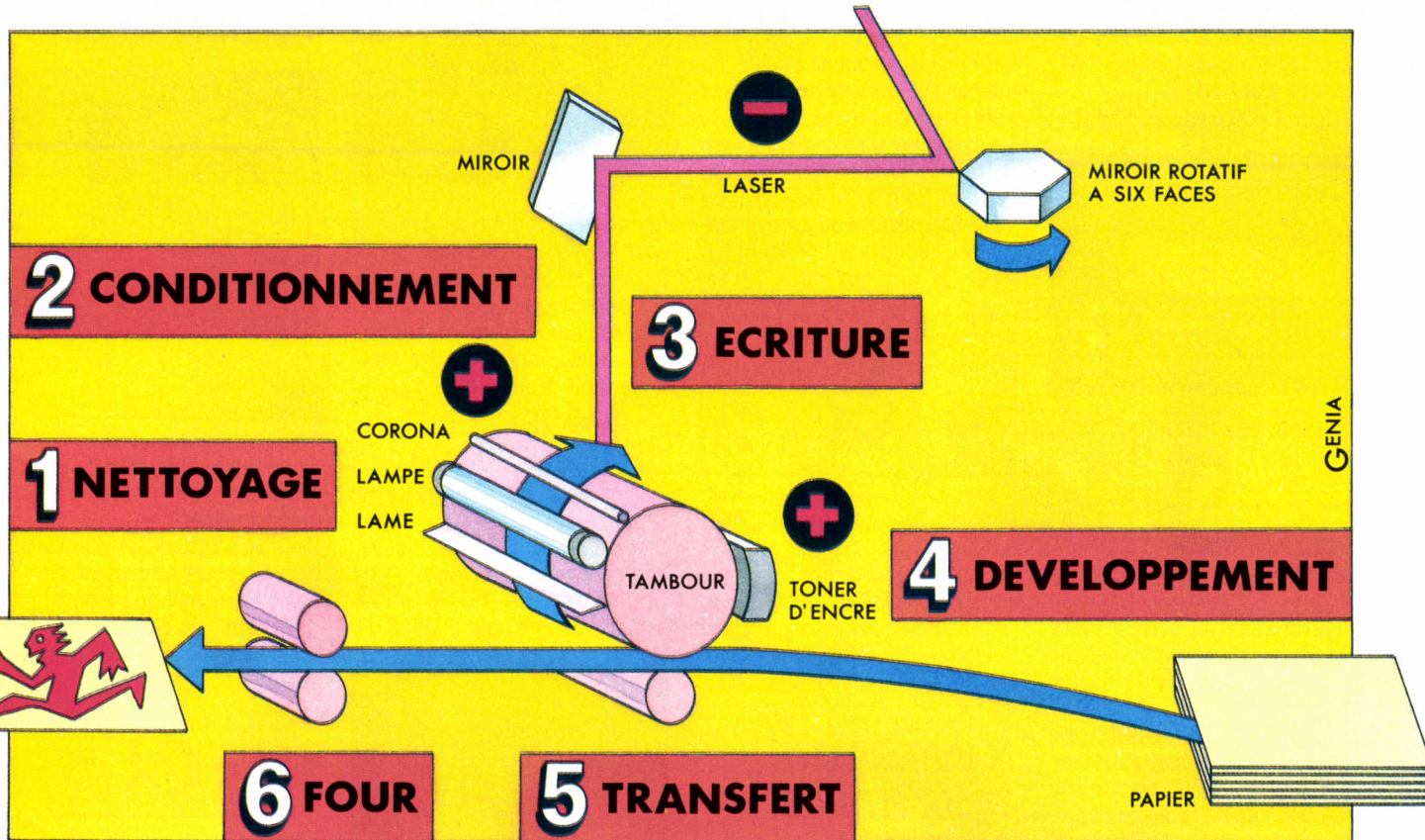
En six phases, le cycle du tambour rotatif situé au cœur d'une imprimante à laser.
