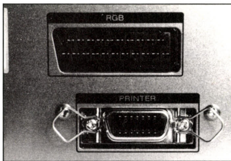
Egalement au dos, la prise PériTel et la sortie pour imprimante Centronics.
