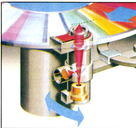
Système de lecture du CD : un prisme dirige le faisceau réfléchi par le disque vers la photodiode.
