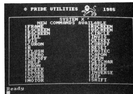
Die Befehlstabelle
