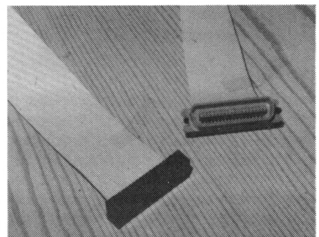
Abb. 4: Das fertige Verbindungskabel für den CPC 6128
