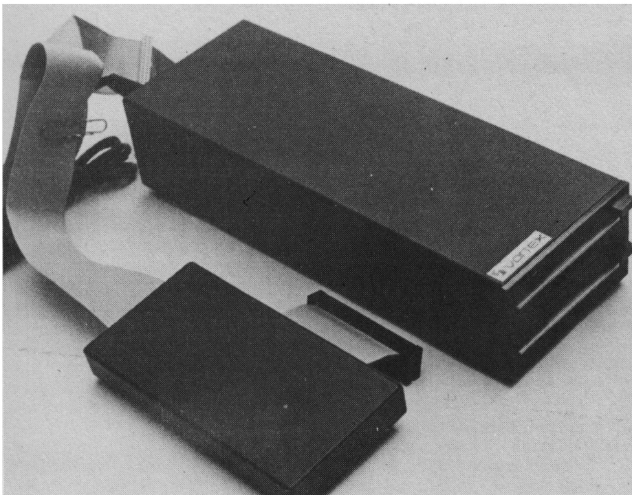
Die neue vortex-Floppy M1D mit Controller. Wie die F1D hat sie komplett 1,4 MByte.
