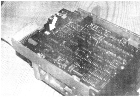
Abb. 5: Die Schalter zum Einstellen der Laufwerksnummer
