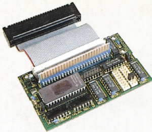
X-Modul in Standardausführung (Abb. ohne Gehäuse)
