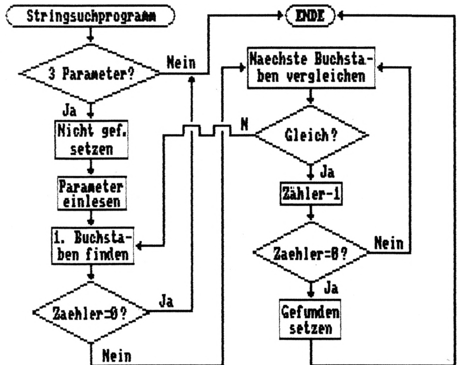
Abbildung 1: Flußdiagramm für das Stringsuch-Programm
