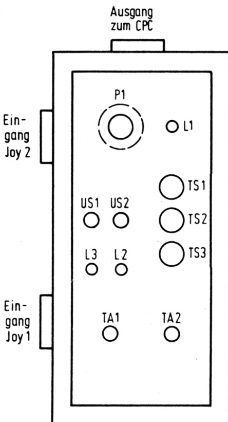
Schema des fertig montierten Y-Switches in der Draufsicht. P1 ist der Regler für die Geschwindigkeit des Dauerfeuers.
