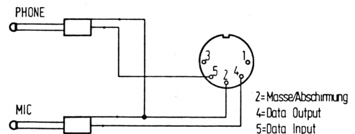
Über Kopfhörer- und Mikrofonanschluß
