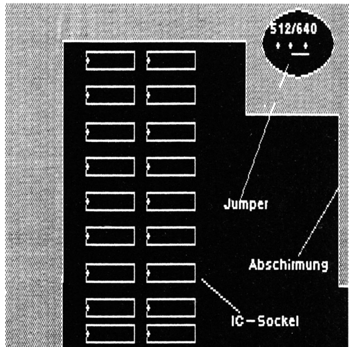
So liegen die 18 IC-Sockel auf der Platine des PC 1512
