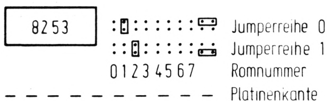
Bild 1 zeigt die Verbindung der Jumper mittels Plastikstecker
