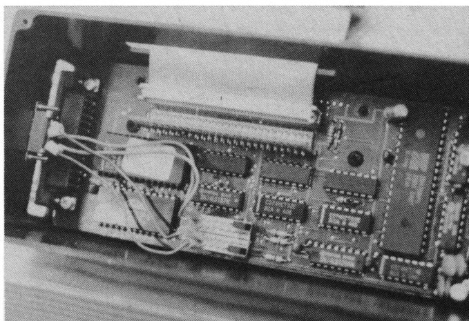
Bild 2: Die Plastikstecker werden durch Kabelverbindungen zum Schalter ersetzt
