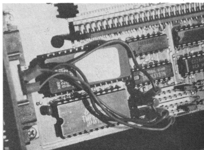
Bild 3: Die Steckkontakte sollten mit Isolierschlauch abgesichert werden
