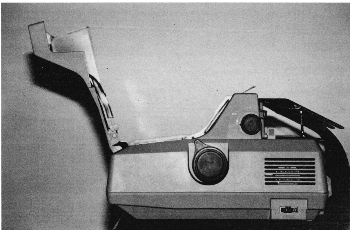
Der P6 (hier mit bidirektionalem Traktor) ist gut von oben her zugänglich
