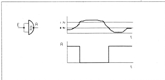
Bild 7: Schmitt-Trigger, Schaltzeichen und Signalverlauf
