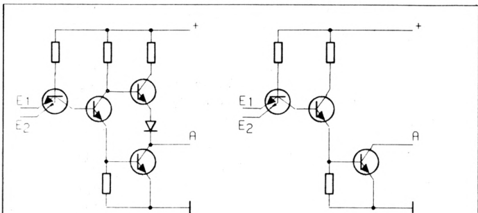
Bild 5a: Aufbau eines TTL-Gatters
