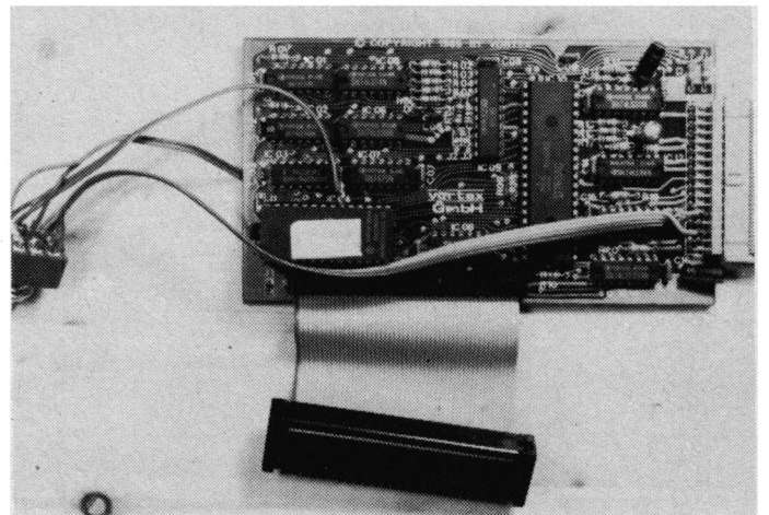
Bild 1: Der vortex-Controller (Oberseite) mit den aufgelöteten Anschlüssen
