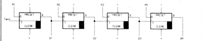
Bild 3d: 4-Bit-Zähler mit D-Flipflops
