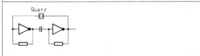
Bild 8: Schaltung eines einfachen Quarzoszillators
