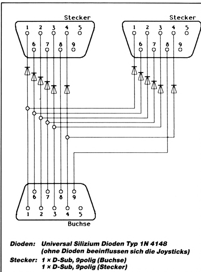
Abb. 1: Anschluß für zwei Standard-Joysticks
