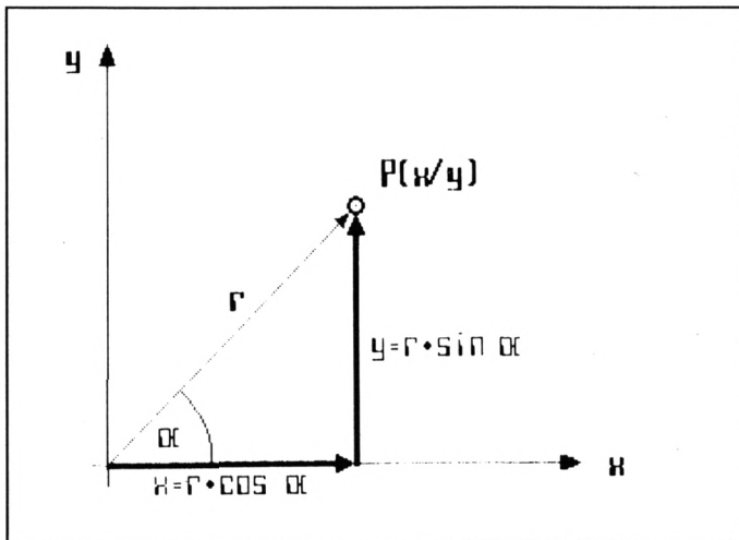
So funktioniert die Berechnung der Kreispunkte mit den Winkelfunktionen
