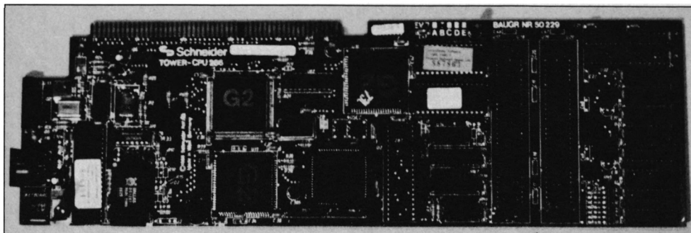
Die Fassungen U29-U32 nehmen die neuen RAM-Chips auf
