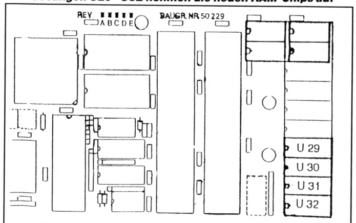
Die Fassungen U29-U32 nehmen die neuen RAM-Chips auf
