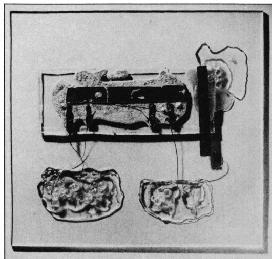
Von der ersten integrierten Schaltung bis zur Produktion der 4-MByte-Chips reicht das Spektrum der Schau.
