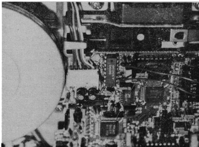
Das Foto zeigt die bei uns durchgeführte Modifikation zur Umschaltung zwischen 40 und 80 Spuren
