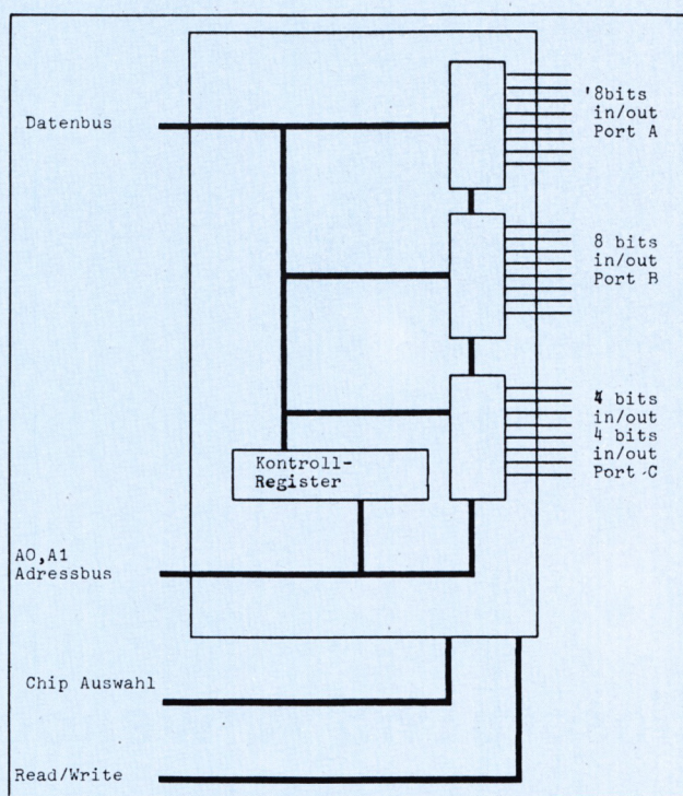
Der D-8255 Ein-/Ausgabe Chip
