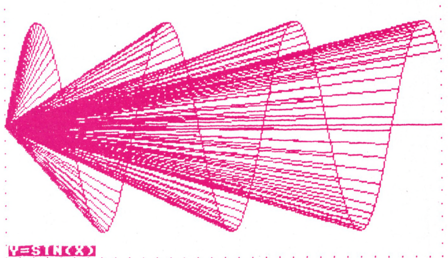
Drei-dimensionale Sinusfunktion, dargestellt im Koordinatensystem
