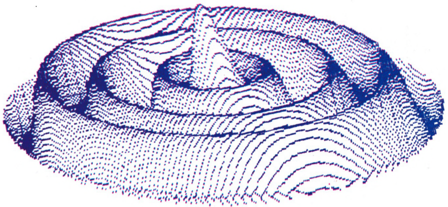
Drei-dimensionale Sinusfunktion in räumlicher Darstellung
