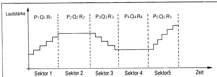
Abbildung III: Lautstärken-Hüllkurve
