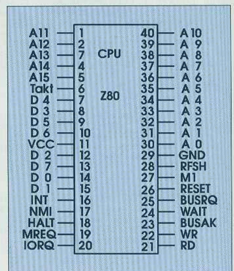
Die CPU Z80
