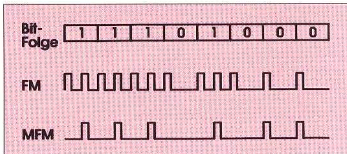
Oben: Das MFM-Verfahren ermöglicht gegenüber dem älteren FM-Verfahren die doppelte Aufzeichnungsdichte Links: Die Aufteilung der Diskette in Spuren und Sektoren Unten: Um die Vorgänge bei der Speicherung zu verdeutlichen, schreiben wir hier den Buchstaben S auf die Diskette
