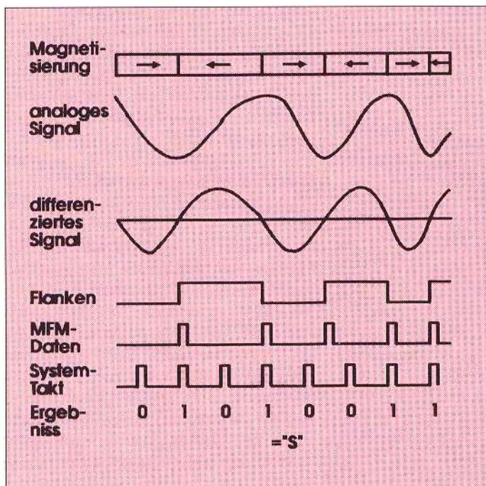
Ein Byte wird von der Diskette gelesen – der Buchstabe S. Mit jedem Impuls des Arbeitstakts wird ein Bit übernommen. Vorher muß aber noch das analoge Signal vom Lesekopf in eine rechteckige Impulsform gebracht werden
