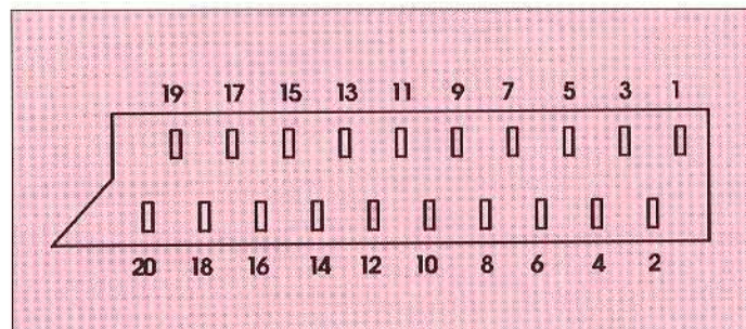
Die Pinbelegung eines SCART-Steckers für den Anschluß an einen Videorekorder
