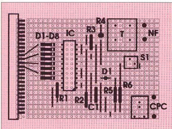
Die Anordnung der Bauelemente auf der Leiterplatte
