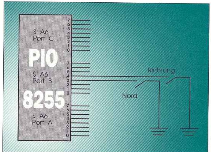
Abb. 3: Einmal aufgebaut, läßt sich die Meßanlage einfach an die PIO anschließen
