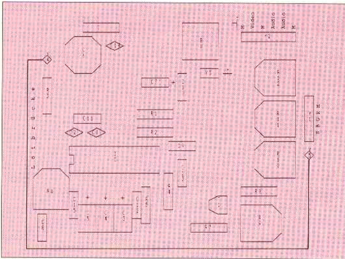
Der Bestückungsplan, von der Teilleseite aus gesehen. Beachten Sie die Lötbrücke, die über die ganze Platine hinweg führt! Wenn man vergißt, sie einzulöten, funktioniert die Schaltung nicht
