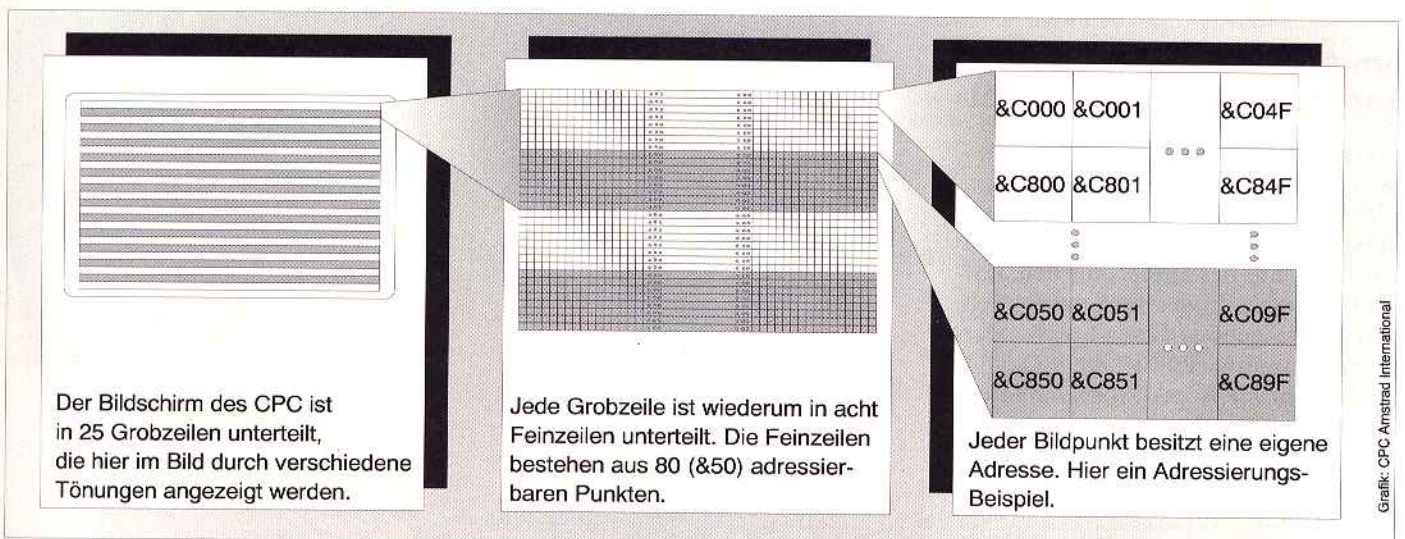
Der Bildschirmspeicheraufbau des CPC
