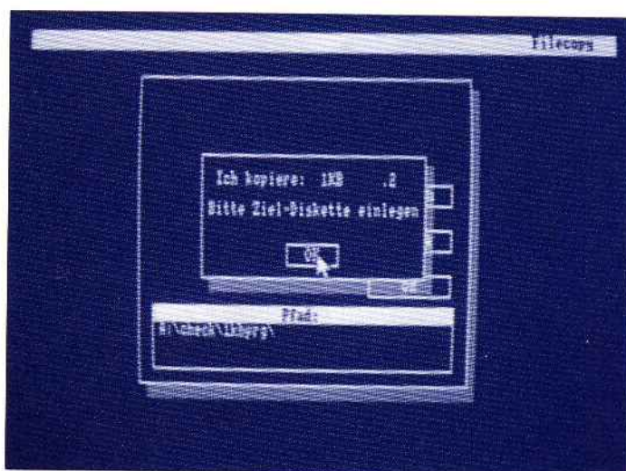
Das Dateien-Kopierprogramm
