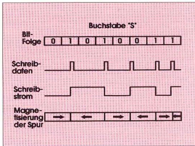
Oben: Das MFM-Verfahren ermöglicht gegenüber dem älteren FM-Verfahren die doppelte Aufzeichnungsdichte Links: Die Aufteilung der Diskette in Spuren und Sektoren Unten: Um die Vorgänge bei der Speicherung zu verdeutlichen, schreiben wir hier den Buchstaben S auf die Diskette
