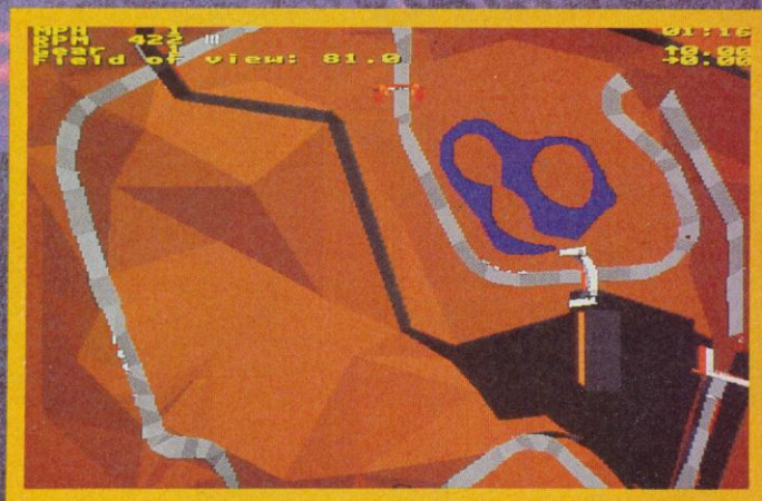
Die Strecke aus der Satellitensicht
