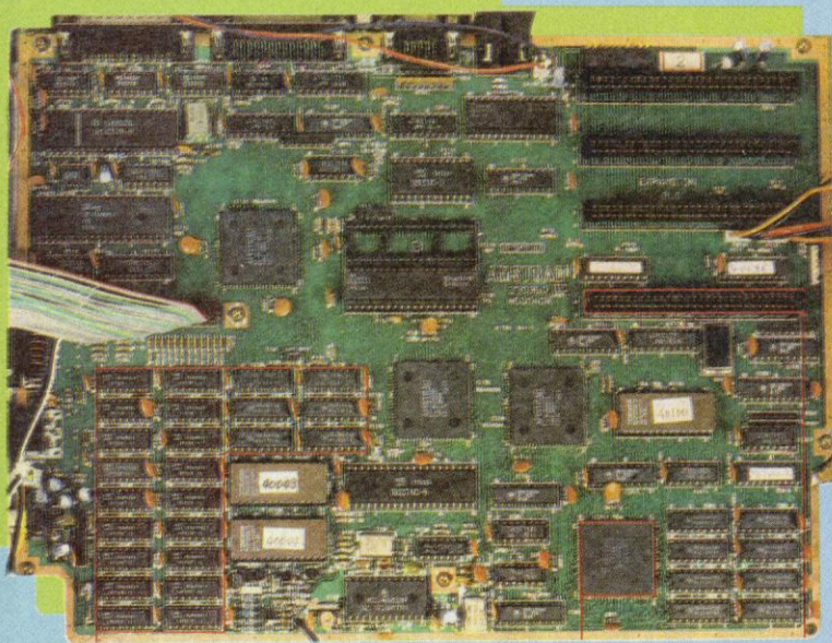
Die Traumplatine des Schneider 1640 in der Draufsicht
