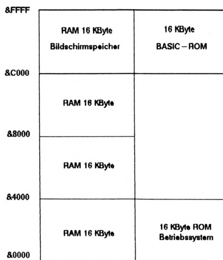
Bild 1: Speicher des CPC 446
