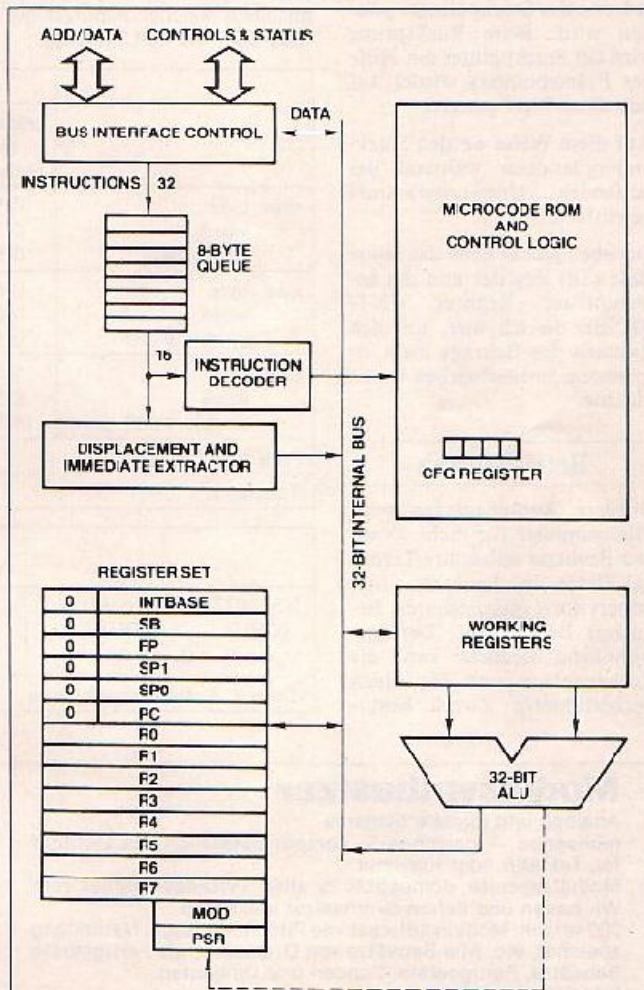
Bild 9. Interne Architektur des 32032
