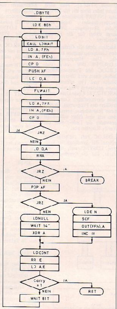
Bild 6. Flußdiagramm für LDBYTE
