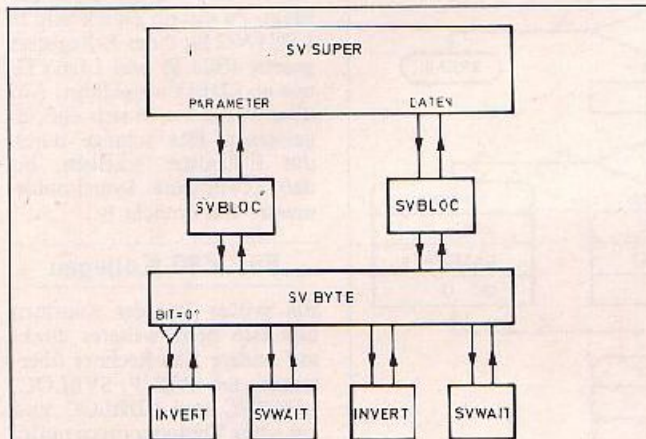
Bild 3. Die SAVE-Routinen
