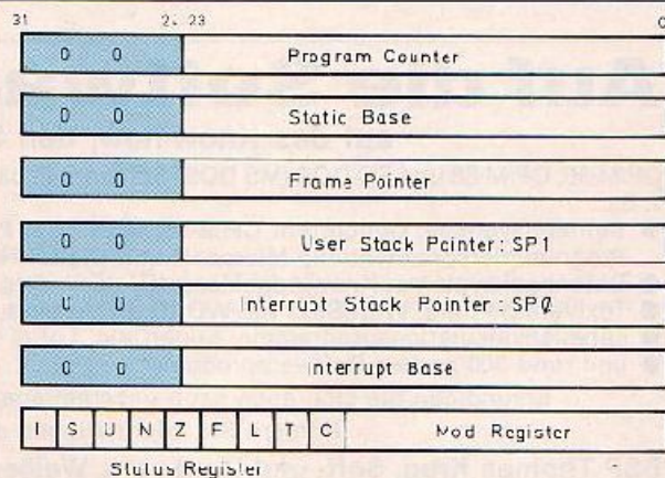
Bild 10. Die fest zugeordneten Register
