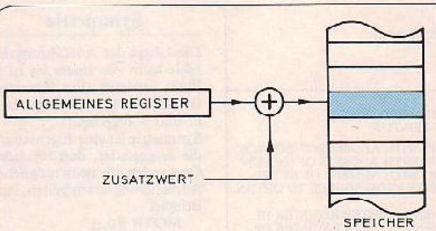
Bild 4. Register-relative Adressierung mit Zusatzwert (Offset)
