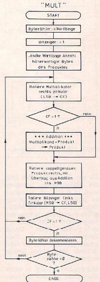
Bild 2. Ablaufplan der Multiplikation
