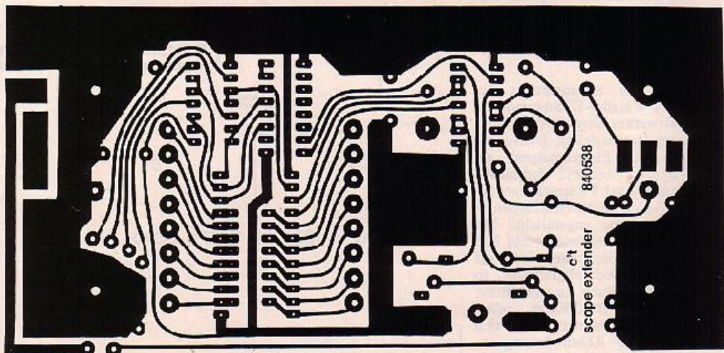
Bild 5. Platinenlayout. Für den Einbau in das Verobox-Gehäuse sollte die Platine auf das Maß 72,4 x 148 mm zugeschnitten werden.
