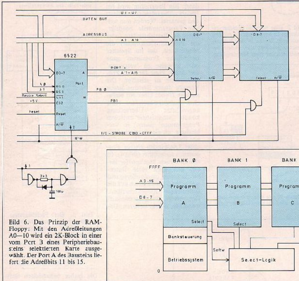
Bild 7. Das Prinzip der Bankumschaltung: Eine Selektlogik übernimmt die physikalische Umschaltung. Die Banksteuerung als Teil des Betriebssystems dient als Schnittstelle zur Selektlogik und verwaltet die einzelnen Speicherseiten.
