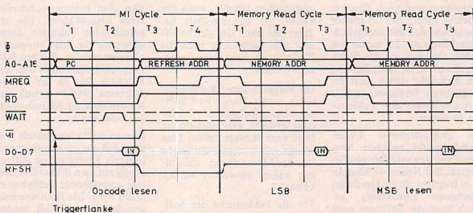
Bild 1. Impulssdiagramm zum Programm TEST 1. Gezeigt ist ein OPCODE Ladezyklus, gefolgt von zwei RAM-Zugriffen. Getriggert wird auf die fallende Flanke von MI. Die Signale können dann auf den zwei Kanälen wiedergegeben werden.
