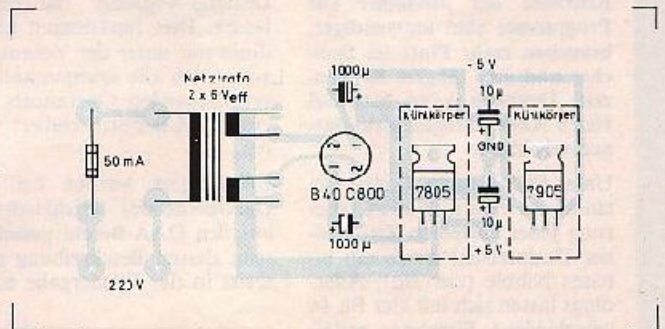
Bild 7. Vorschlag für ein geeignetes Netzteil
