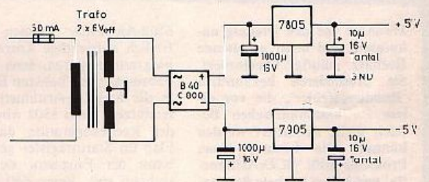
Bild 7. Vorschlag für ein geeignetes Netzteil
