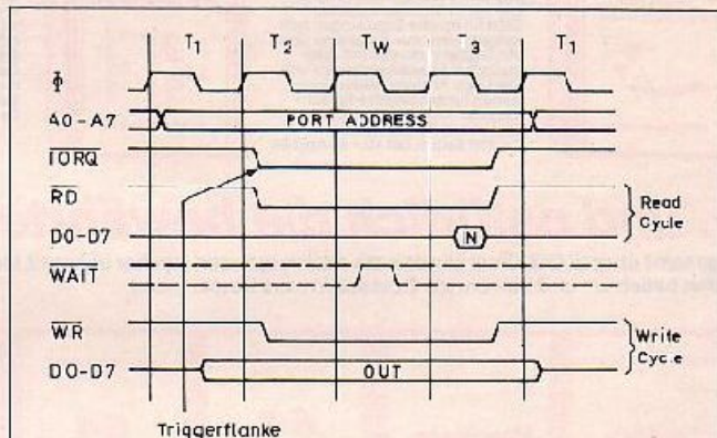
Bild 3. Impulsverläufe bei I/O-Zugriff. Die Triggereung erfolgt auf der fallenden Flanke des IORQ. Die Daten können innerhalb der nächsten 3 Taktzyklen beobachtet werden.
