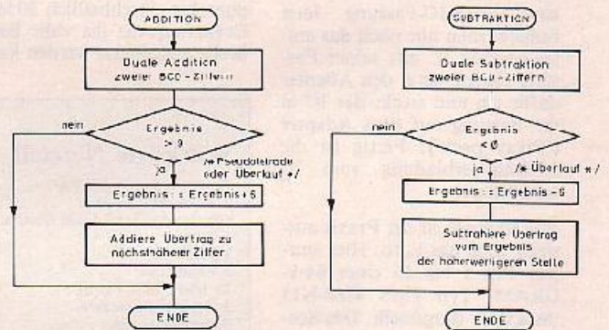
Bild 2. Dezimaler Abgleich
