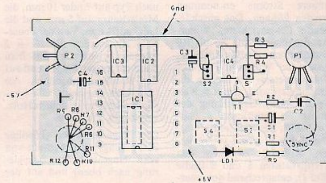
Bild 4. Bestückungsplan. Die Bauteile werden auf der Leiterbahnseite aufgelötet.
