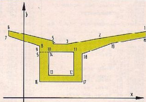
Bild 8: Spannungsermittlung an einem Brückenprofil
