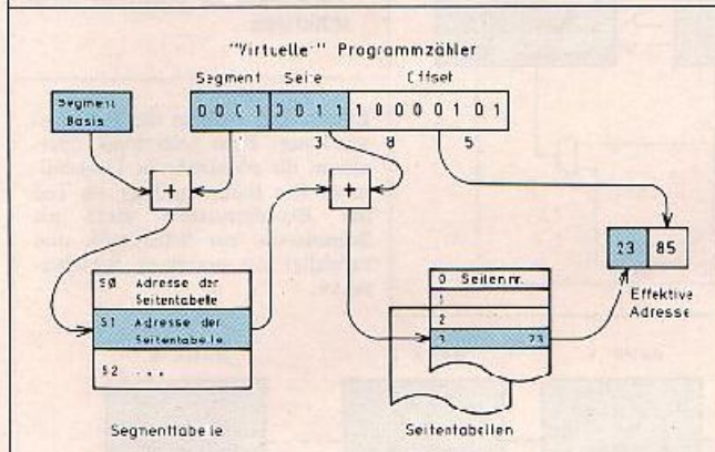
Bild 3. Umsetzung einer 'virtuellen' Adresse in eine effektive Speicheradresse. Durch Segment- und Seitentabelle wird die physikalische Lage der Speicherstelle variabel.
