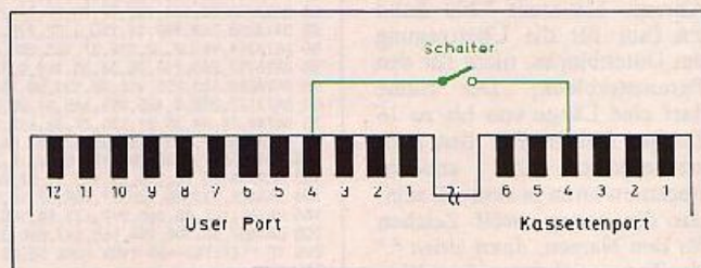
Bild 1. SuperTape-'Hardware'
