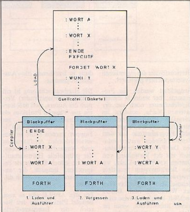
Bild 4. Die Ausführung von Programmen in FORTH. Das Wort FORTH an den richtigen Stelle ermöglicht die Ausführung von umfangreichen Programmen in einem vergleichsweise kleinen Speicher.
