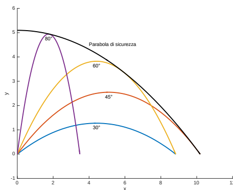
Figura 4 Traiettorie del proiettile al variare di m
