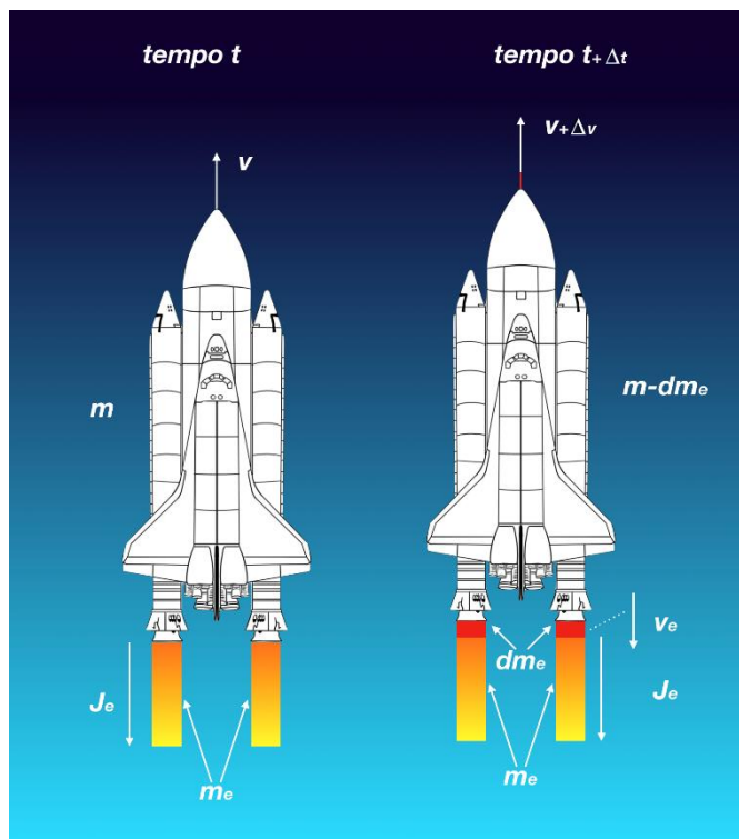
Fig. 4: Il principio di azione / reazione
