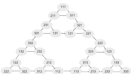
Figura 7. Grafo associato al problema delle Torri di Hanoi.
