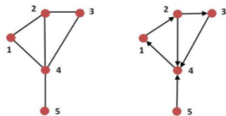
Figura 3. Grafo non orientato (a sinistra) e orientato (a destra).
