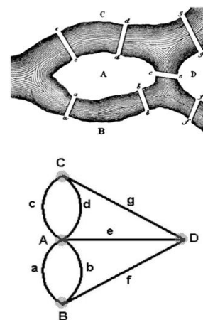
Figura 2. Grafo associato al problema dei 7 ponti.
