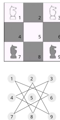
Figura 4. Il problema dei 4 cavalli.
