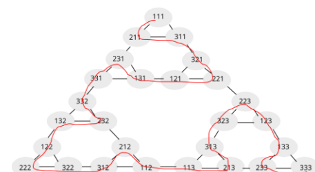
Figura 8. Cammino Hamiltoniano per le Torri di Hanoi.
