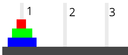
Figura 5. Le torri di Hanoi.
