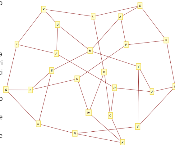
Figura 9. Grafo per il gioco della tabella 5 \times 5 .
