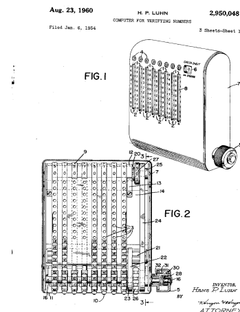
Figura 1. Dispositivo portatile brevettato da Luhn.
