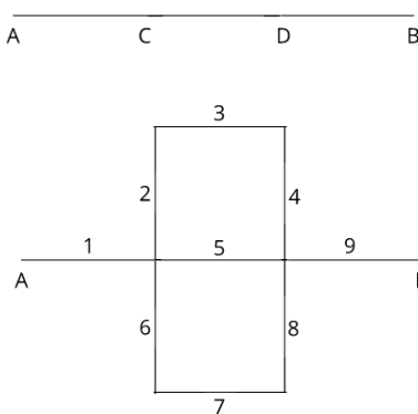
Figura 2. Costruzione della curva di Peano
