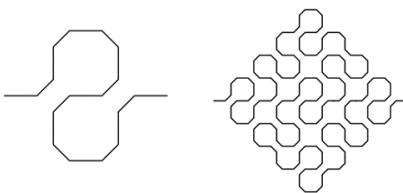
Figura 3. Due iterazioni del procedimento di Peano.
