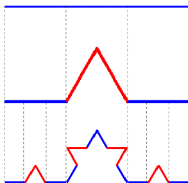
Figura 5. Due iterazioni della curva di Koch
