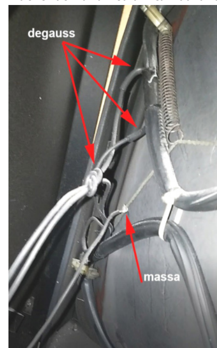
Fig.6 - Collegamento della gabbia di smagnetizzazione attorno al tubo catodico
