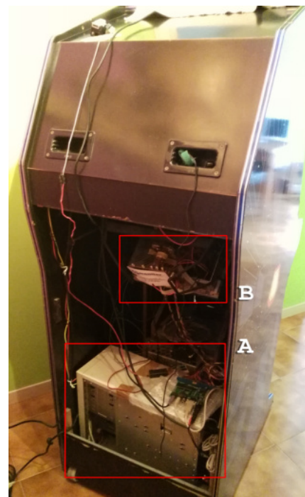
Fig. 2 - Riquadro A: computer con scheda JammASD sopra; Riquadro B: retro del tubo catodico con scheda di controllo -
