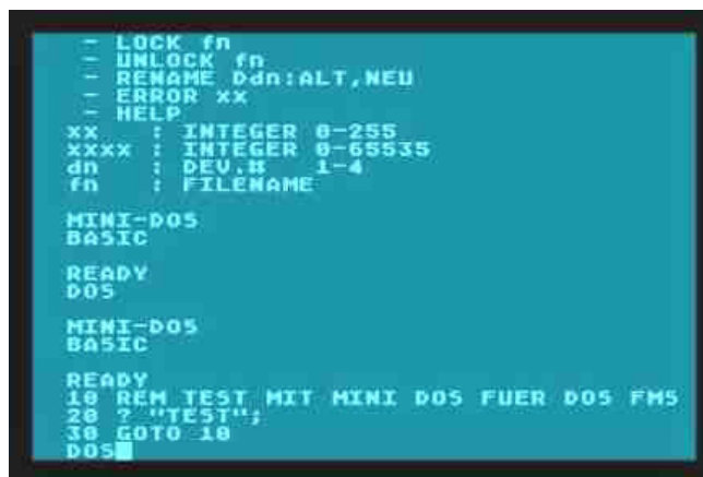
Fig.6 - Schermata d'uso del MiniDOS per Atari 8-bit
