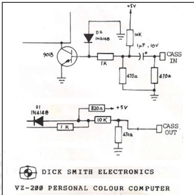
Esempio di interfaccia a cassette semplificata degli home computer: un transistor, due diodi e qualche altro componente (Dick Smith VZ200 / Laser 210).
