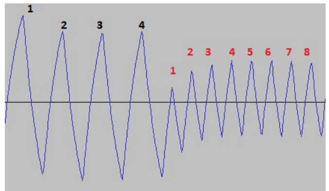
Il segnale audio di un bit "0" seguito da un bit "1" - a causa della particolare circuiteria adottata nella scheda LX.385 dello Z80NE, il segnale non è un'onda sinusoidale e neanche un'onda quadra, ma un'onda "quasi" triangolare.
