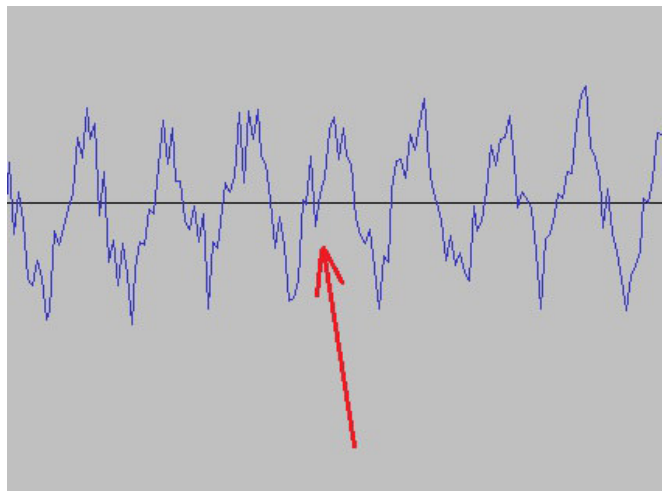
Nella foto: il rumore causa un falso passaggio per lo zero dell'onda.
