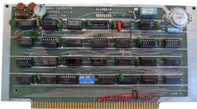
La scheda Tarbell Tape Interface per bus S-100 (1976)
