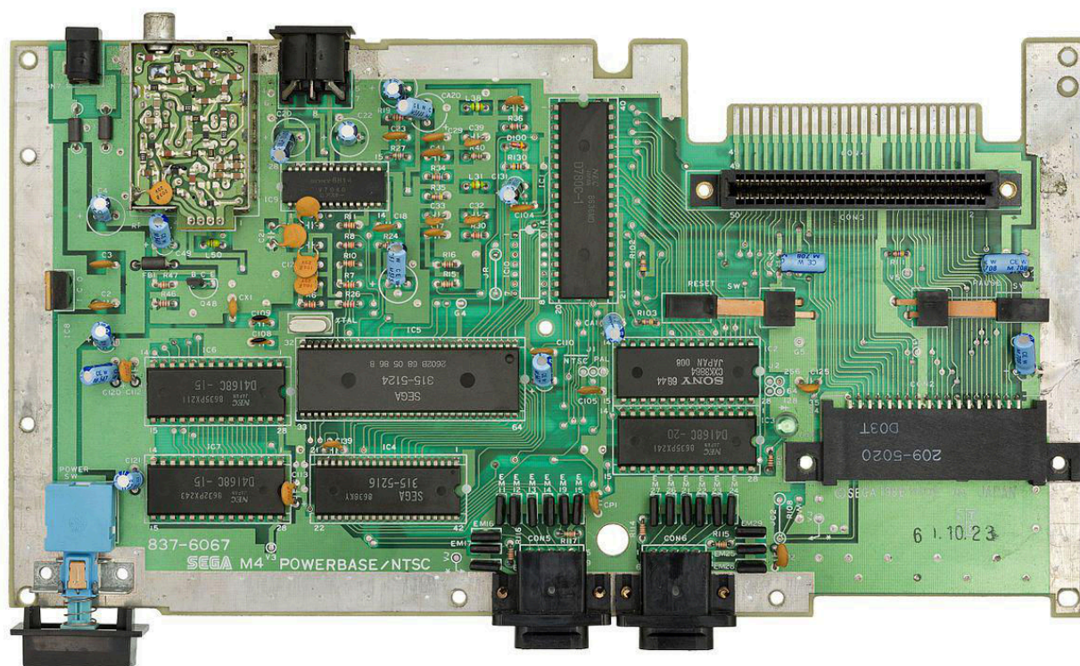
Fig. 3 - Scheda madre del Sega Master System: si notano la CPU Z80 (il chip centrale posto verticalmente), il VDP (il grosso chip leggermente a sinistra rispetto al centro). Sul lato destro la porta Sega Card (in basso) e quella per le cartucce (in alto) (foto: Evan-Amos – fonte: Wikimedia Commons)
