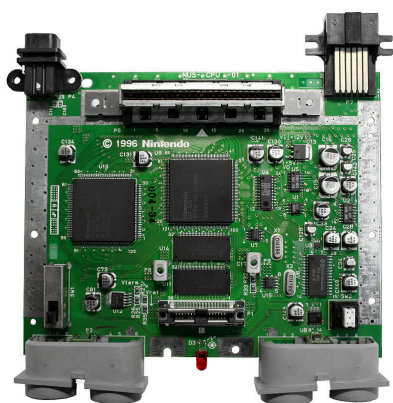
La scheda madre del Nintendo 64 con la CPU, l'RCP (il Reality Co-Processor) e la RDRAM
