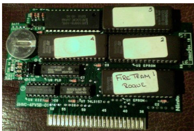
Fig. 5 - Il primo prototipo della cartuccia
