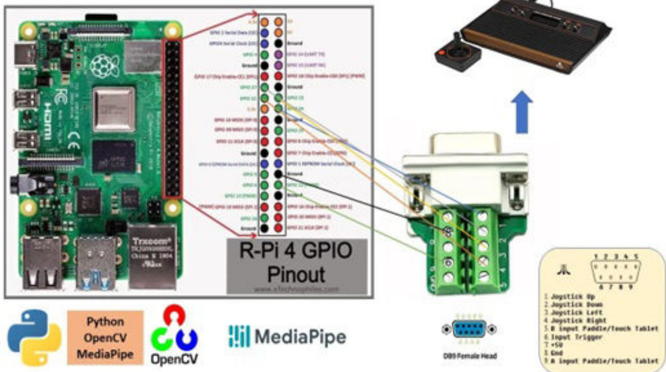
Fig. 1 - Lo schema di collegamento
