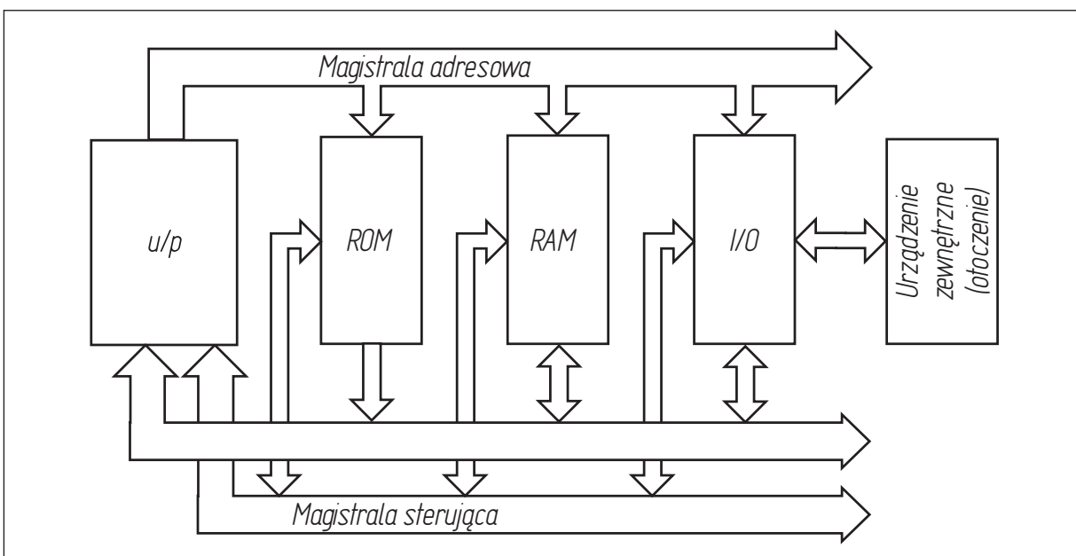
Schemat blokowy komputera
