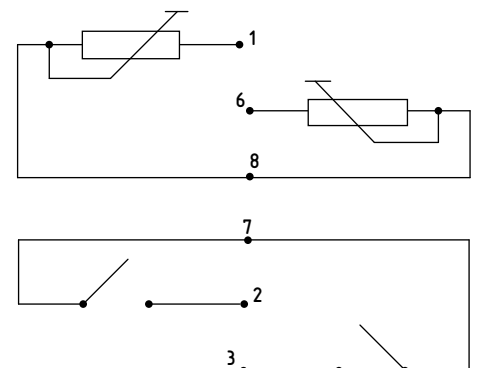
Rys. 2. Schemat elektryczny zespołu wiośetek.
