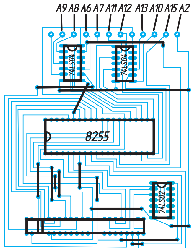
Rys. 3 Schemat montażowy, widok od strony elementów
