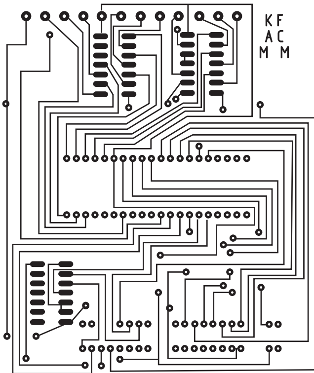
Rys. 2 Płytkowa drukowana interface'u skala 1:1
