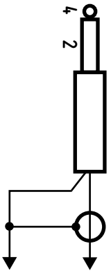
Rys. 1 Wtyk słuchawkowy
