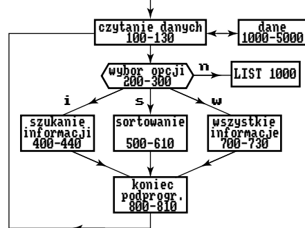
Rys. 1. Schemat blokowy działania programu bazy danych.
