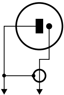
Rys. 1 Wtyk głośnikowy
