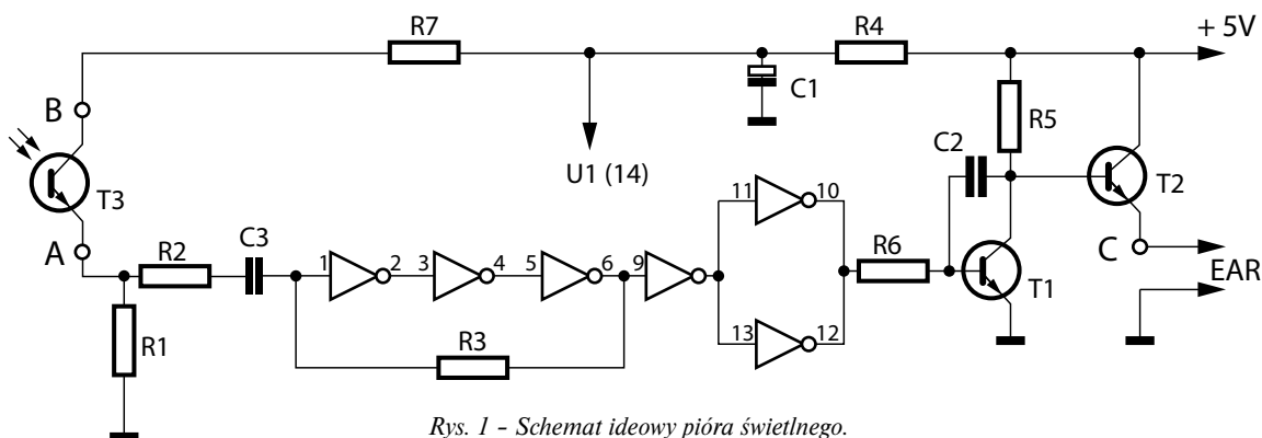
Rys. 1 - Schemat ideowy pióra świetlnego.
