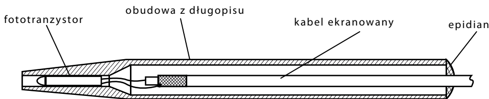
Rys. 2 - Konstrukcja mechaniczna pióra.
