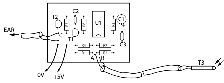
Rys. 4 - Rozmieszczenie elementów na płytce.
