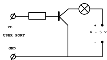
Rys. 4 Schemat podłączenia układu żarówki do pojedynczej szyny USER PORTU. Przy podłączeniu ośmiu takich układów zasilanie może być wspólne.
