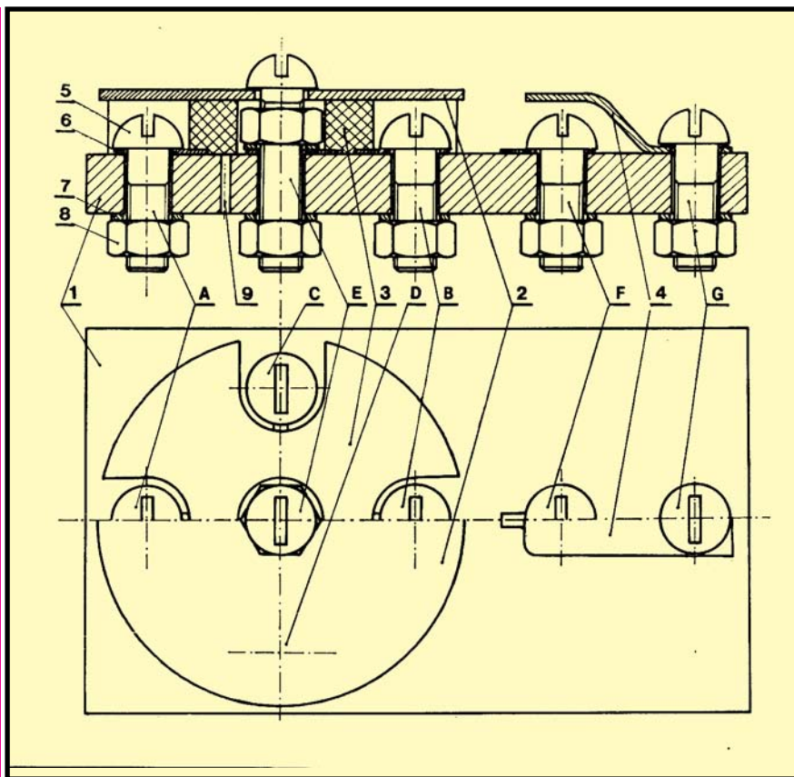
Rys. 1. Konstrukcja manipulatora: 1 – podstawa, 2 – blaszka, 3 – gąbka, 4 – styk sprężysty „fire”, 5 – wkręty z łbami okrągłymi (7 sztuk), 6 podkładka stykowa (7 sztuk), 7 – podkładka zwykła (8 sztuk), nakrętka ośmiokątna (8 sztuk), 9 – otwór na przewody elektryczne.
