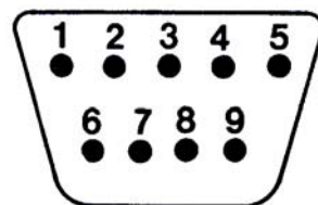
Rys. 4. Wtyczka Eltra 881, widok od strony połączeń lutowniczych.
