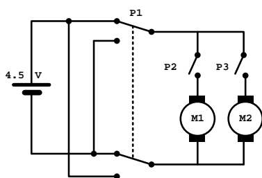
Rys. 1 Schemat układu sterującego samochodem.
