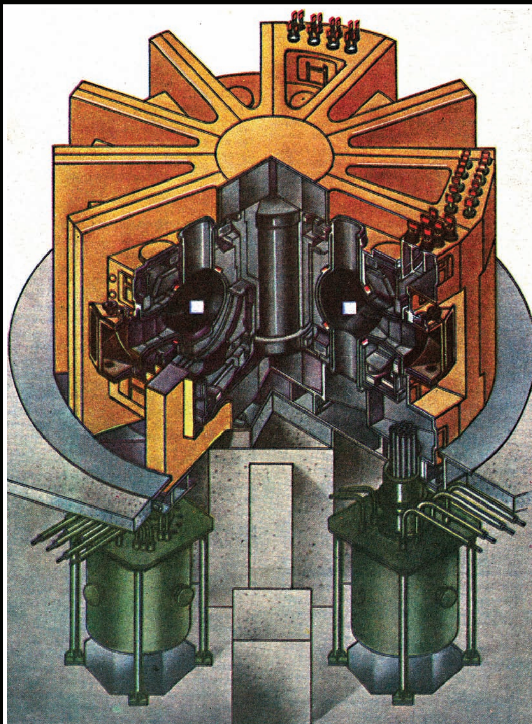
OGÓLNY WIDOK I PRZEKRÓJ TOKAMAKA T-15. PRZEKRÓJ „OBWARZANKA” CZYLI KOMORY ROBOCZEJ, W KTÓREJ ZNAJDOWAĆ SIĘ BĘDZIE PLAZMA, OZNAČA BIAŁY KWADRACIK.
