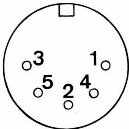
Schemat złącza Composite Video
