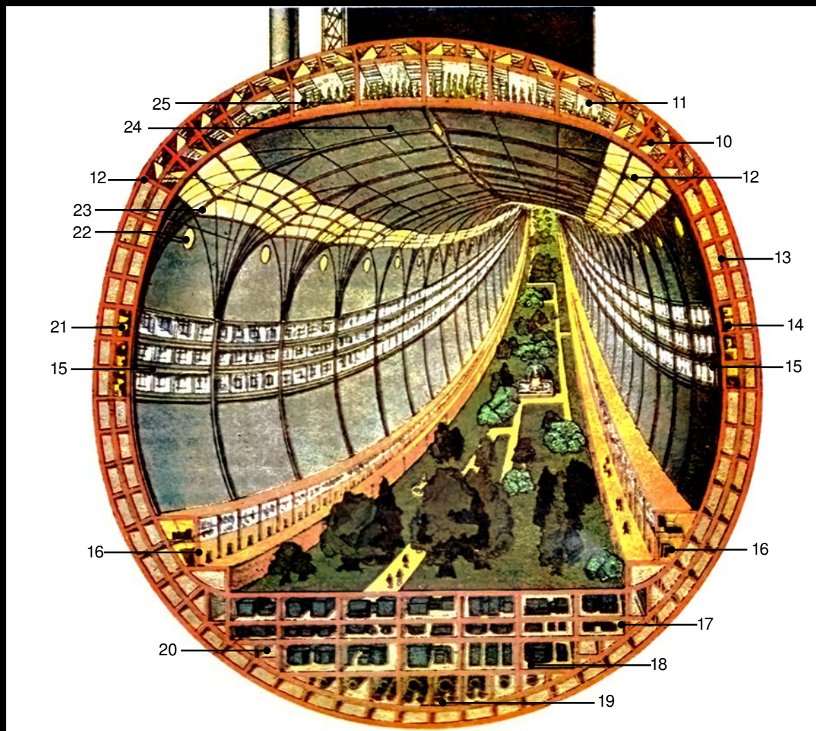
Przekrój-poprzeczny kosmicznego miasta typu toroidalnego. 10. Lustra oświetlające okna głównej przestrzeni życiowej miasta. 11. Lustro oświetlające strefę rolniczą. 12. Okna głównej przestrzeni życiowej miasta. 13. Bloki konstrukcyjne toroidu. 14. Aparatura w wewnętrznych sekcjach ścian. 15. Balkony. 16. Główna strefa mieszkalna miasta z kawiarniami i sklepami na parterze. 17. Schrony awaryjne. 18. Strefa przemysłowa. 19. Podstawowe rurociągi i kable systemu zasilania i łączności. 20. Magazyny. 21. Zaplecze systemu sterowania. 22. Sztuczne oświetlenie. 23. Konstrukcje szkieletu wewnętrznego. 24. Dach (znajduje się w odległości 113 metrów od „ziemi”). 25. Strefa rolnicza.
