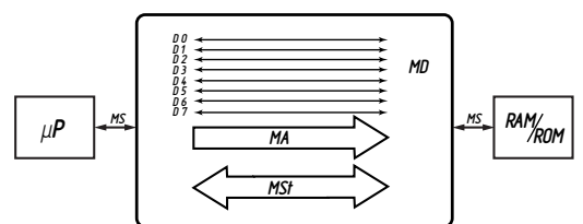
Rys. 3 MD: magistrala danych MA i St: magistrala adresowa i sterująca
