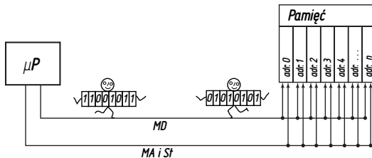
Rys. 2 MD: magistrala danych MA: magistrala adresowa MSi: magistrala sterująca MS: magistrala systemowa DO..., DI: przewody danych od 0÷7
