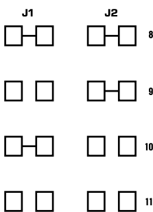
Rys. 3. Kombinacje połączeń złączy J1 i J2 i odpowiadające im numery urządzenia.
