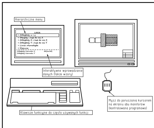
Wprowadzanie danych w systemie stacji graficznej WS10.
