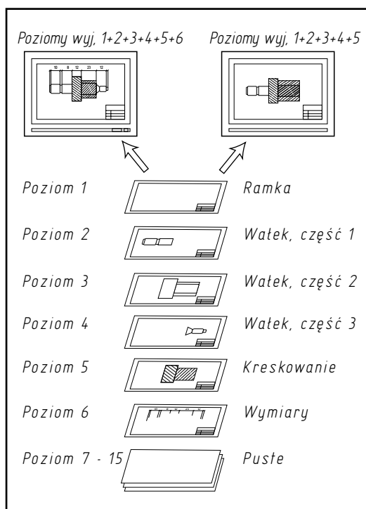
Technika warstwowa tworzenia rysunków.
