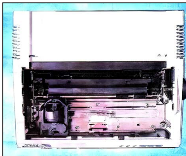
Widoczna głowica z taśmą barwiącą oraz elementy mechaniczne.
