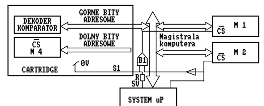
Rys. 2 Schemat blokowy podłączenia cartridge'a z odłączeniem pamięci wewnętrznej.
