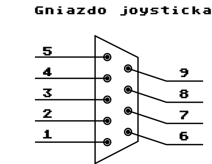
Rys. 1. Połączenie PORT A z gniazdami joysticków.
