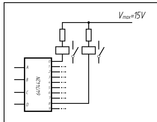
Rys. 3 — jest to w zasadzie taki sam układ jak opisany wyżej. Różnica polega jedynie na zastosowaniu dekodera z obwodem otwartego kolektora w stopniu wyjściowym. Dzięki temu możliwe jest dołączenie przekaźników na inne napięcie niż 5V, jednak nie wyższe niż 15V. Do styków przekaźników można dołączyć na przykład żarówki sieciowe.
