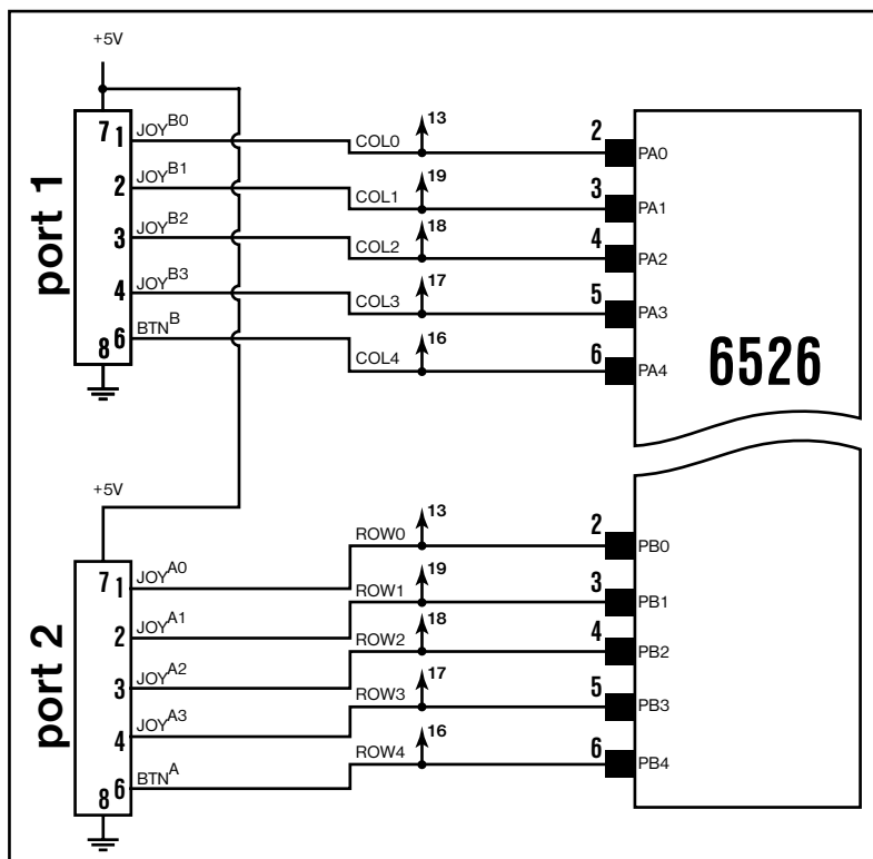
Rys. 2. Połączenie portów drążków z układem CIA — Commodore 64. Strzałki wskazują połączenie linii ze złączem klawiatury. Wartości cewek nieznanne. Wartości kondensatorów CA0-CA3 i CB0-CB3 = 100 pikofaradów, C71 = 0,1 mikrofarada.
