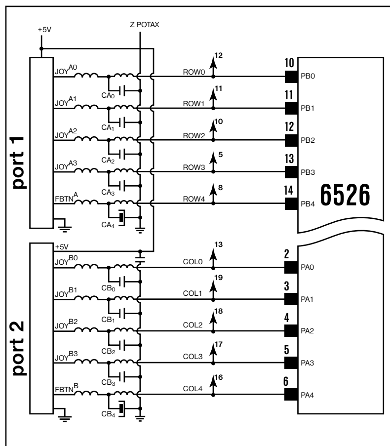
Rys. 1. Połączenie portów drążków z układem CIA — Commodore 128. Strzałki wskazują połączenie linii ze złączem klawiatury.
