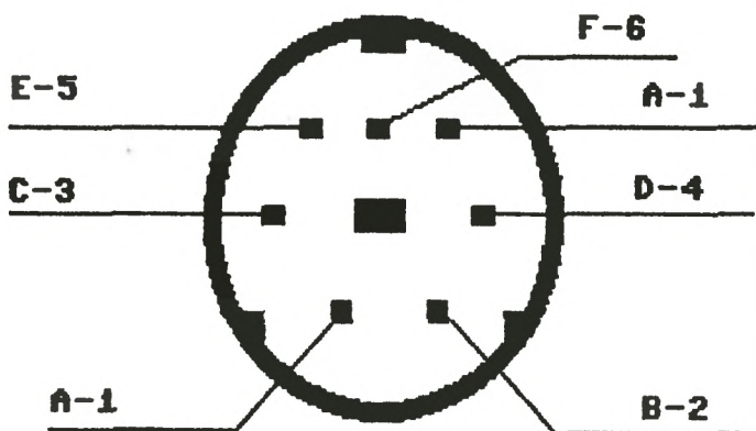
Wtyk magnetofonu 1531 (widok z przodu wtyczki)
